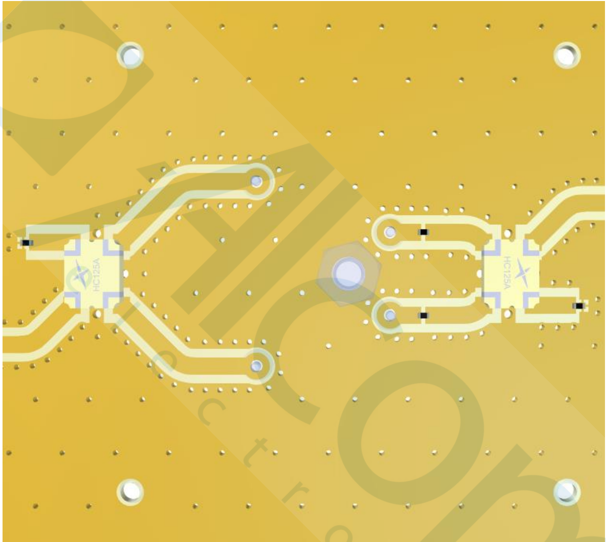
Bottom Side
